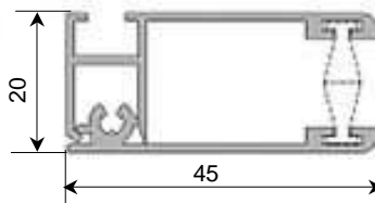
FS 35 x 17,5 FS 45 x 20
