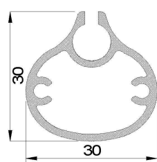
FP 30 x 30 Tropfenform
